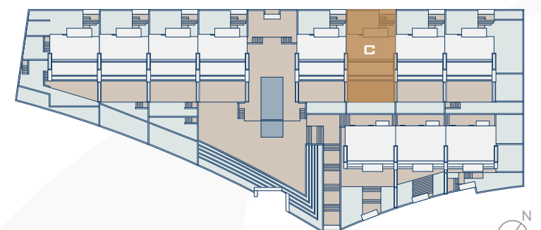
Planta segunda
